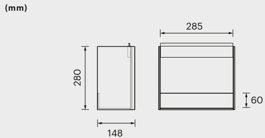
PORTA OGGETTI IN VETRO Vetro fumè e alluminio nero 598800056
