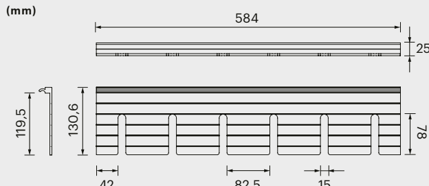
PORTA CALICI Nero 598800042
