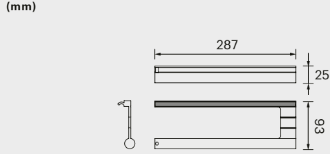
PORTA ROTOLO Nero 598800019
