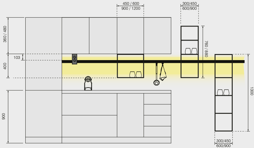
ESEMPIO DI INSTALLAZIONE IN CUCINA (mm)
